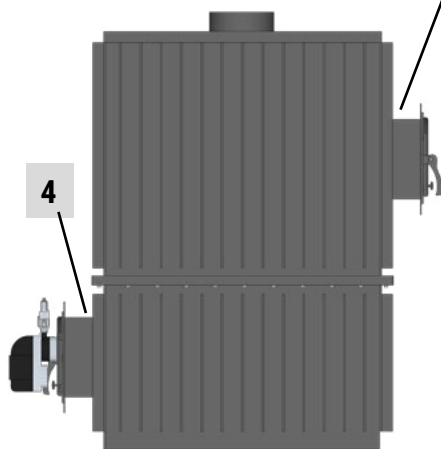
Рис. 1в. Печь «Севастополь -МГТ». Вид сбоку.
