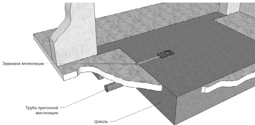
Рис. 4. Фундамент печи с вентиляционным каналом
