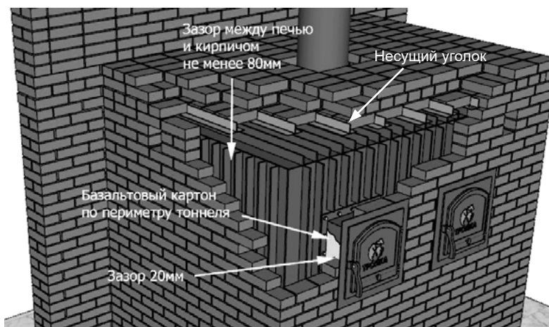
Рис. 5. Обкладка печи кирпичом со стороны каменки
