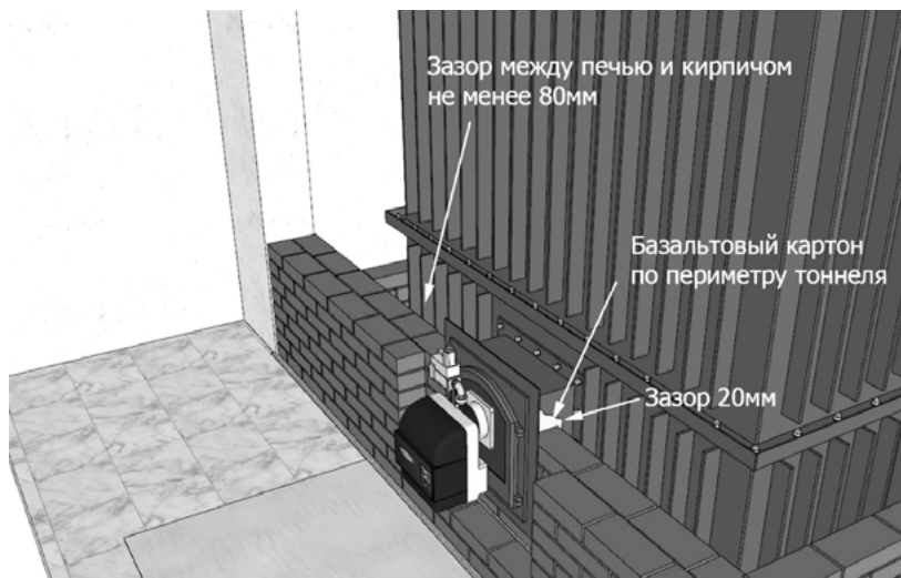
Рис. 6. Обкладка печи кирпичом со стороны горелки
