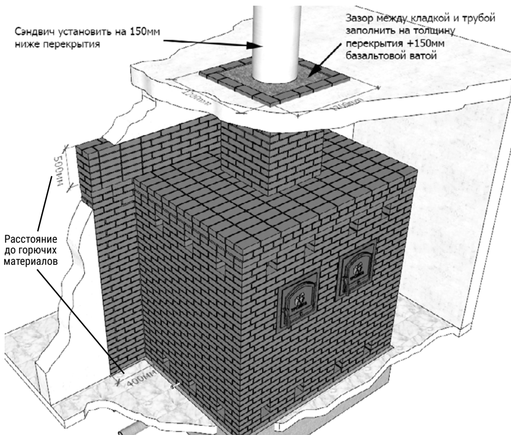
Рис. 8. Проход дымоходом и кирпичной трубой перекрытия.
