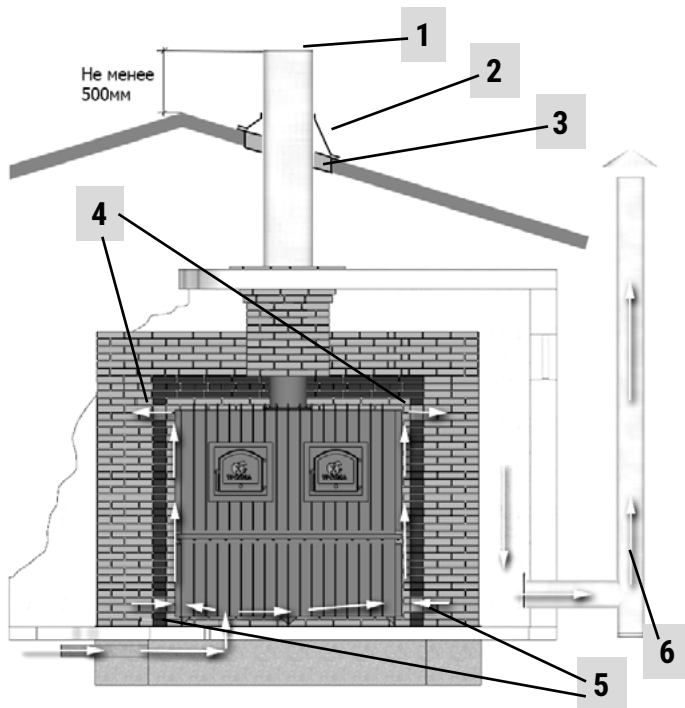
Рис. 7. Циркуляция воздуха
